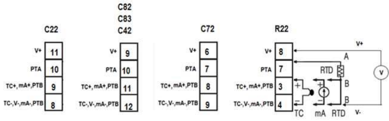
2-25. Sensor Input Wiring
