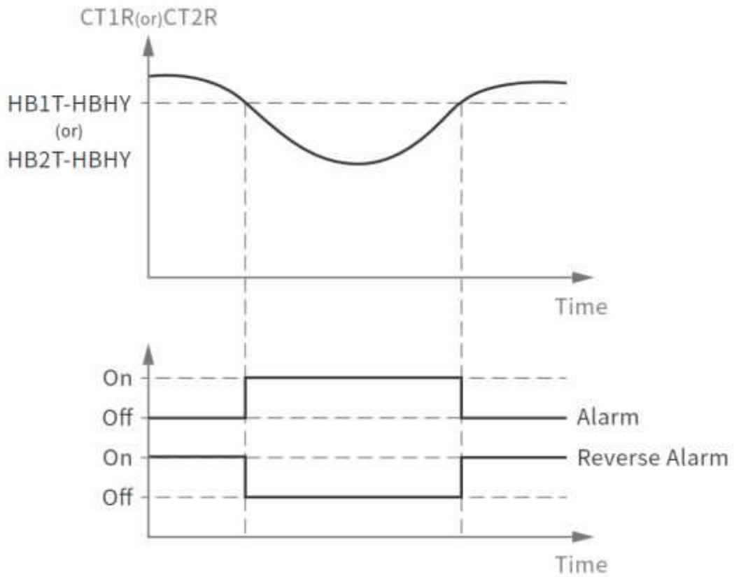
3-11 Heater Break(H.bk)
