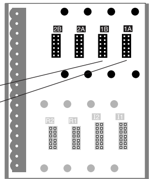
*F1 図1? 出力モジュールのスロットは、後ろから見た場合、コントロールの回路板の上半分にあります。
