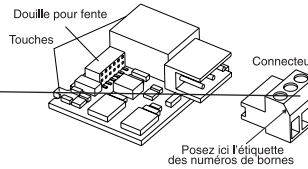
Figure 4 — Retirez le connecteur et mettez à jour l'étiquette avant d'installer le module.
