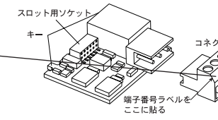
*F4 図4? モジュールを取り付ける前に、コネクタを外してラベルを新しくします。
