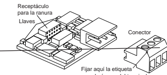
Figura 4 — Desenchufe el conector y actualice la etiqueta antes de instalar el módulo.
