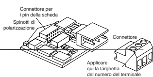
Figura 4 — Prima di installare il modulo, scollegare il connettore e aggiornare la targhetta.
