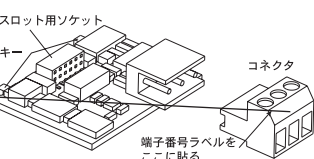
*F4 図4 - モジュールを取り付ける前に、コネクタを外してラベルを新しくします。
