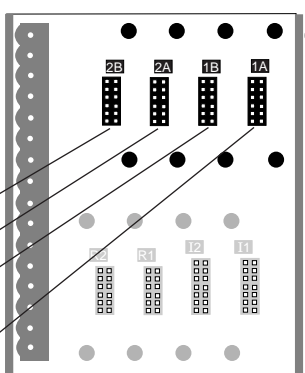
Figura 1 — Las ranuras del módulo de salida del colector abierto se encuentran en la mitad superior de la placa del circuito impreso del controlador (visto desde atrás).
