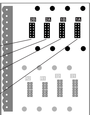
*F1 図1 - 出力モジュールのスロットは、後ろから見た場合、コントローラの回路板の上半分にあります。
